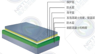
发泡混凝土上人屋面构造图
