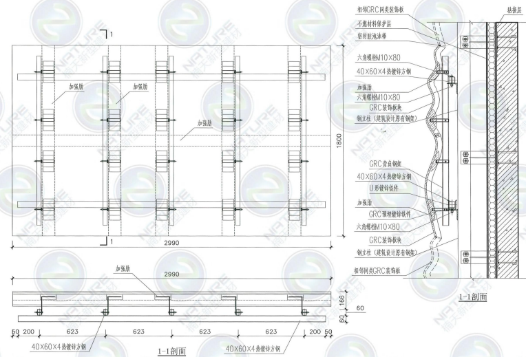
图A.3 GRC有肋框架板大样节点图
